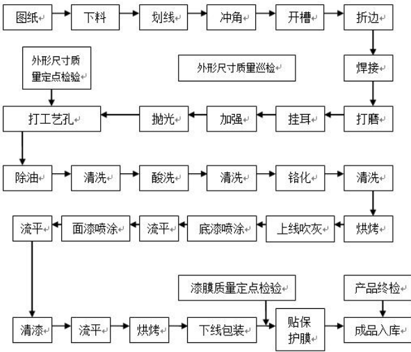
图 3-2-1 铝单板生产工艺流程图
